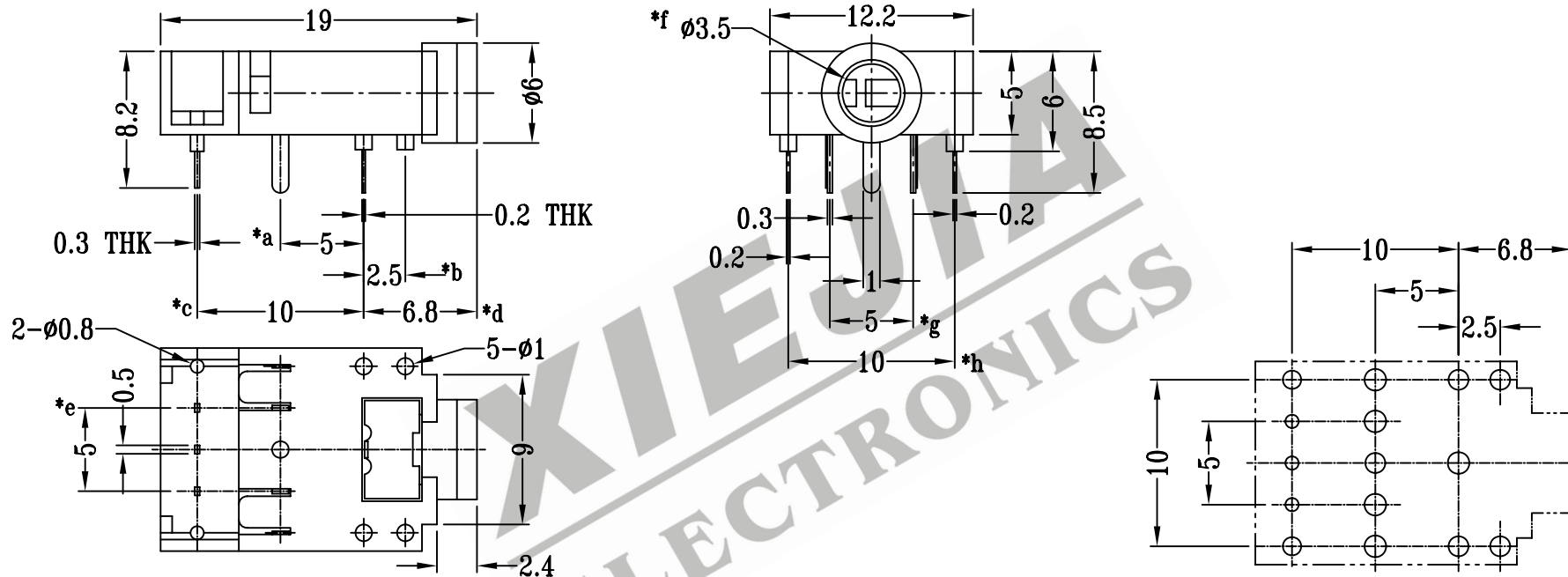
P.C.B LAYOUT
